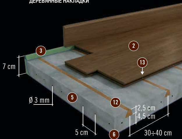
INCHIODATURA SU MAGATELLI IN LEGNO NAILING ON WOODEN LATHS ЗАБИВКА ГВОЗДЯМИ НА ДЕРЕВЯННЫЕ НАКЛАДКИ
