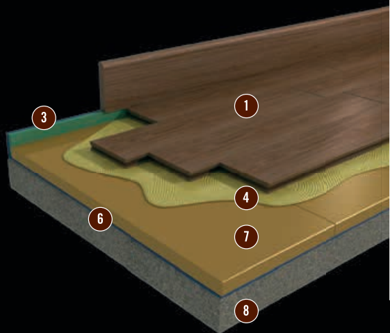
INCOLLAGGIO SU SOTTOFONDO GALLEGGIANTE GLUING ON FLOATING FOUNDATION СКЛЕИВАНИЕ НА ПЛАВАЮЩИЙ ПОДСТИЛАЮЩИЙ СЛОЙ
