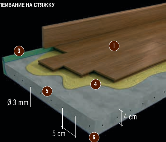
INCOLLAGGIO SU MASSETTO GLUING ON CONCRETE СКЛЕИВАНИЕ НА СТЯЖКУ
